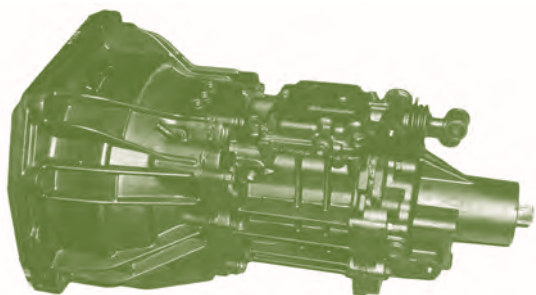
Caja de cambios Suzuki Jimny (modelos hasta 2005)
